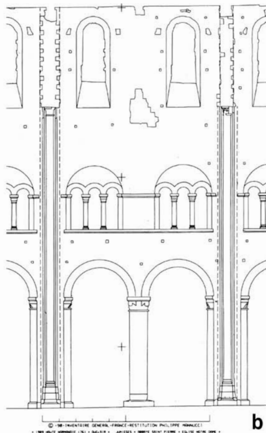
31. a) Modena, Duomo, veduta della parete nord della navata centrale (da Lanfranco e Wiligelmo 1984); b) Jumièges, Notre-Dame, porzione del rilievo fotogrammetrico dell'elevato nord della navata centrale (da MORGANSTERN 1996).
