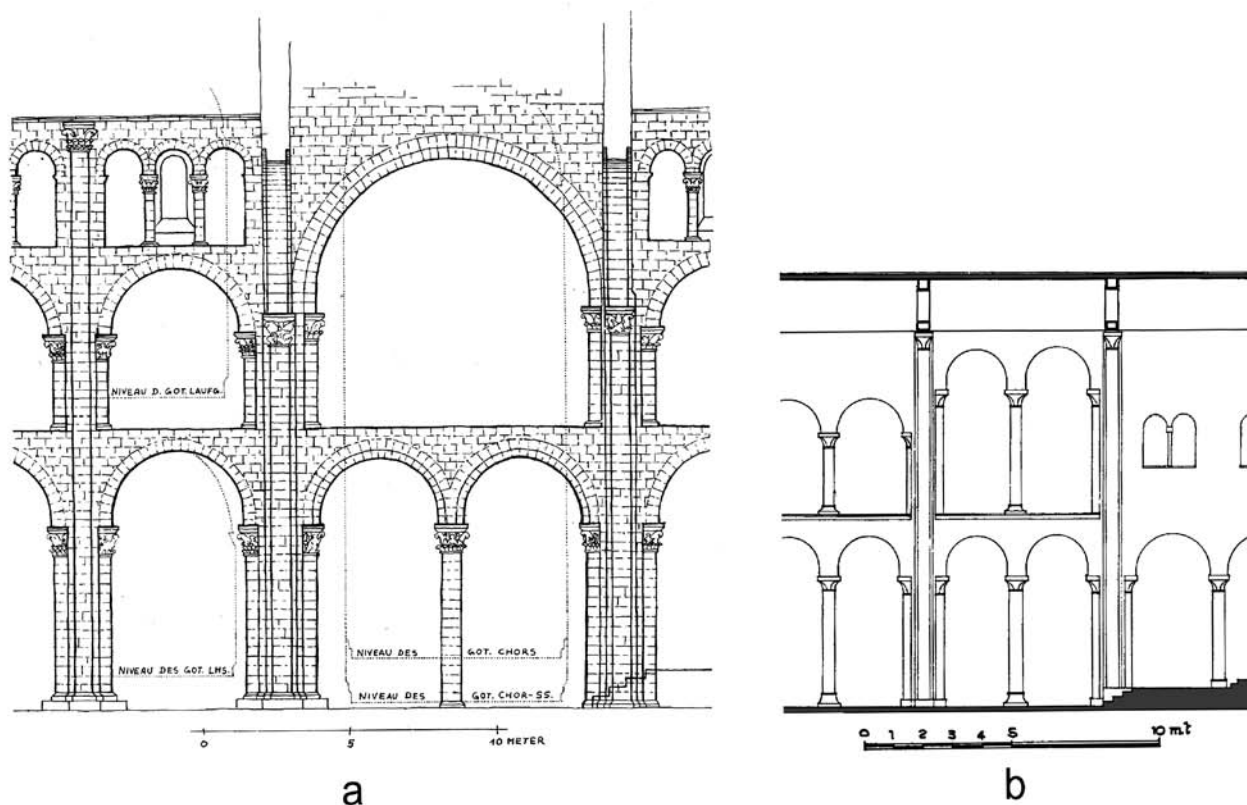
30. a) Bayeux, Notre-Dame, disegno ricostruttivo dell'elevato della navata centrale, campata d'incrocio (da LIESS 1967); b) Verona, San Lorenzo, disegno dell'elevato della navata centrale in corrispondenza del transetto (da ROMANINI 1964). I disegni sono in scala fra loro.
