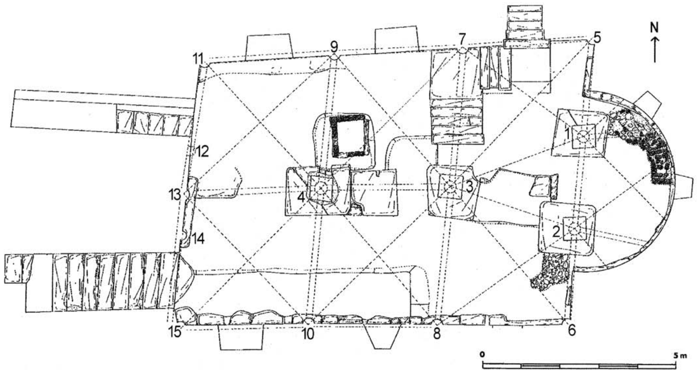
1. Verona, San Benedetto al Monte, pianta (da CAVALIERI MANASSE 2007).
