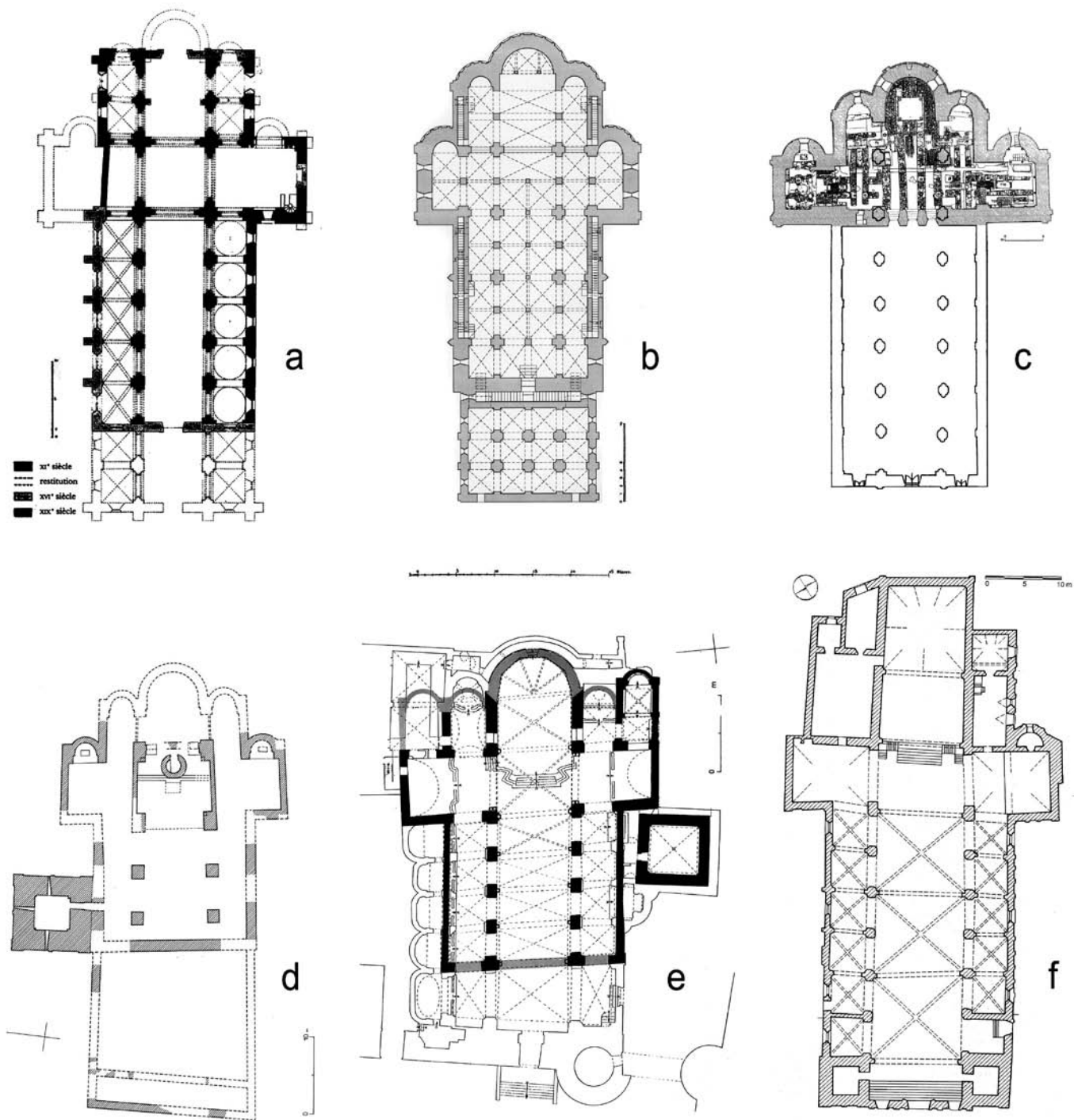
33. a) Bernay, Notre-Dame (da BAYLÉ 1997); b) Verona, San Fermo Maggiore, pianta ricostruttiva della cripta; c) Acqui, Cattedrale (da CROSETTO 2000); d) San Benigno Canavese, San Benigno (da PEJRANI BARICCO 1996); e) Susa, San Giusto (da PEJRANI BARICCO 2002); f) Bobbio, Cattedrale (da SEGAGNI MALACART 1982). Le planimetrie sono in scala fra loro.
