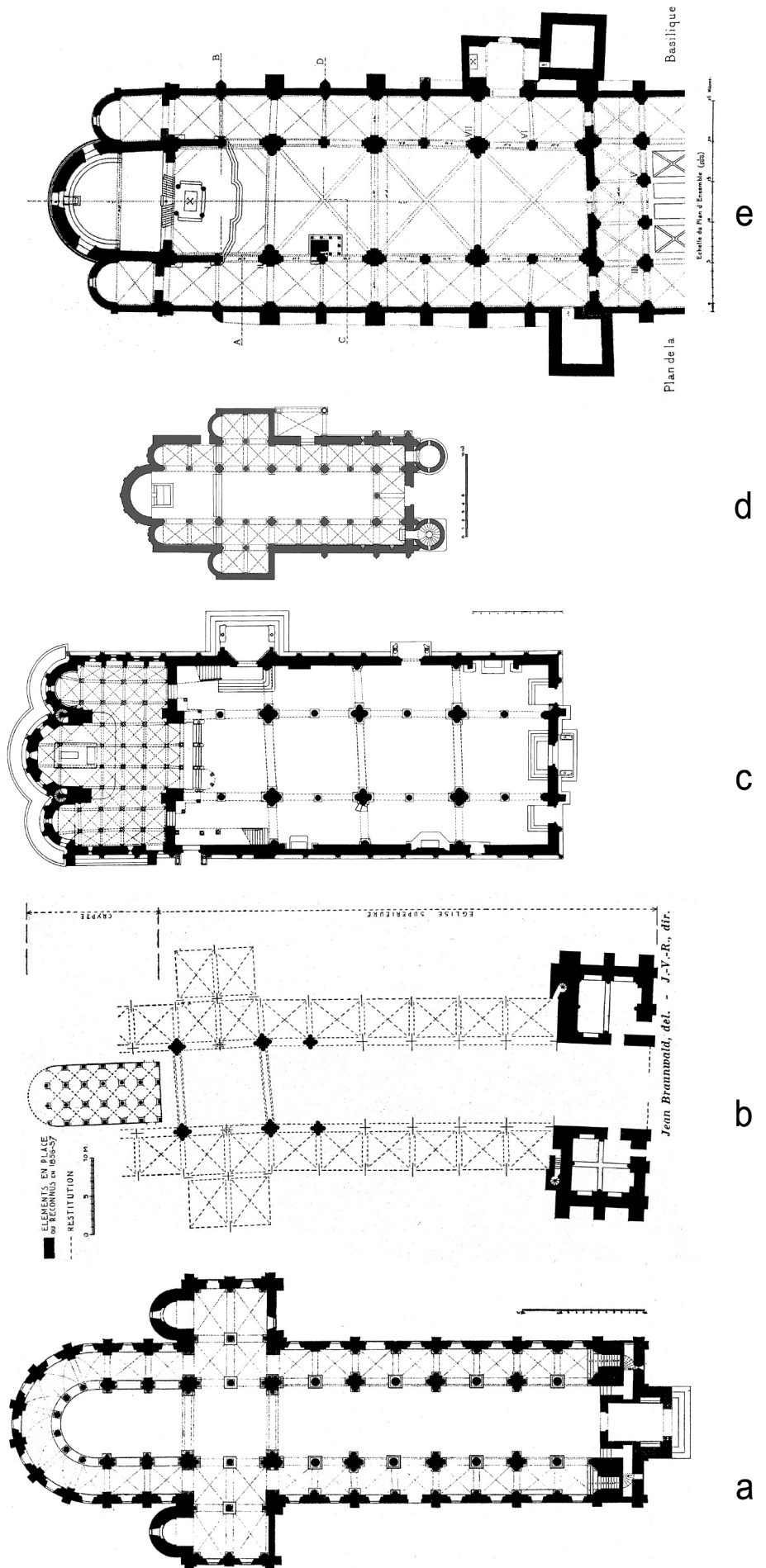
29. a) Jumièges, Notre-Dame (da BAYLÉ 1997); b) Bayeux, Notre-Dame (da VALLE- RY-RADOT 1958); c) Modena, Duomo (da Lanfranco e Wiligermo 1984); d) Verona, San Lorenzo (da ROMANINI 1964); e) Mila- no, Sant'Ambrogio (da DARTEIN 1865- 1882). Le planimetrie sono in scala fra loro.
