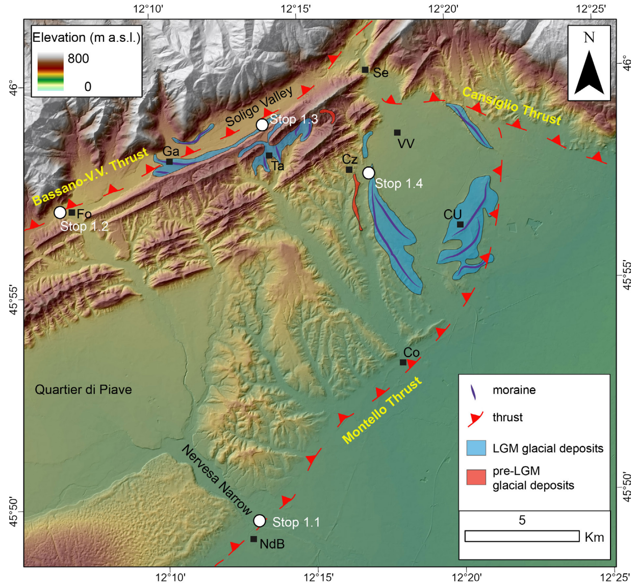
Fig. 5 - Digital elevation model of the Venetian Foothills and piedmont plain with major tectonic features (see Fig. 2). Extent of glacial deposits according to Venco (1963, 1977). Co: Conegliano; CU: Colle Umberto; Cz: Cozzuolo; Fo: Follina; Ga: Gai; NdB: Nervesa della Battaglia; Se: Serravalle; Ta: Tarzo; VV: Vittorio Veneto.
