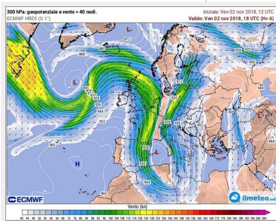
Fig. 3 - Principali campi di vento della tempesta Vaia (da: ilmeteo.net - https://www.ilmeteo.net/ ).
