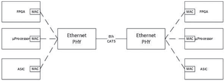
Fig. 3.35. Ethernet subsystem.
