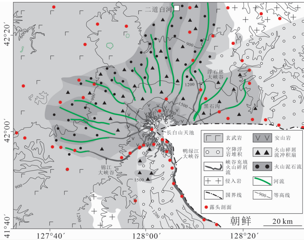
图4 长白山千年大喷发火山碎屑堆积物平面分布特征
