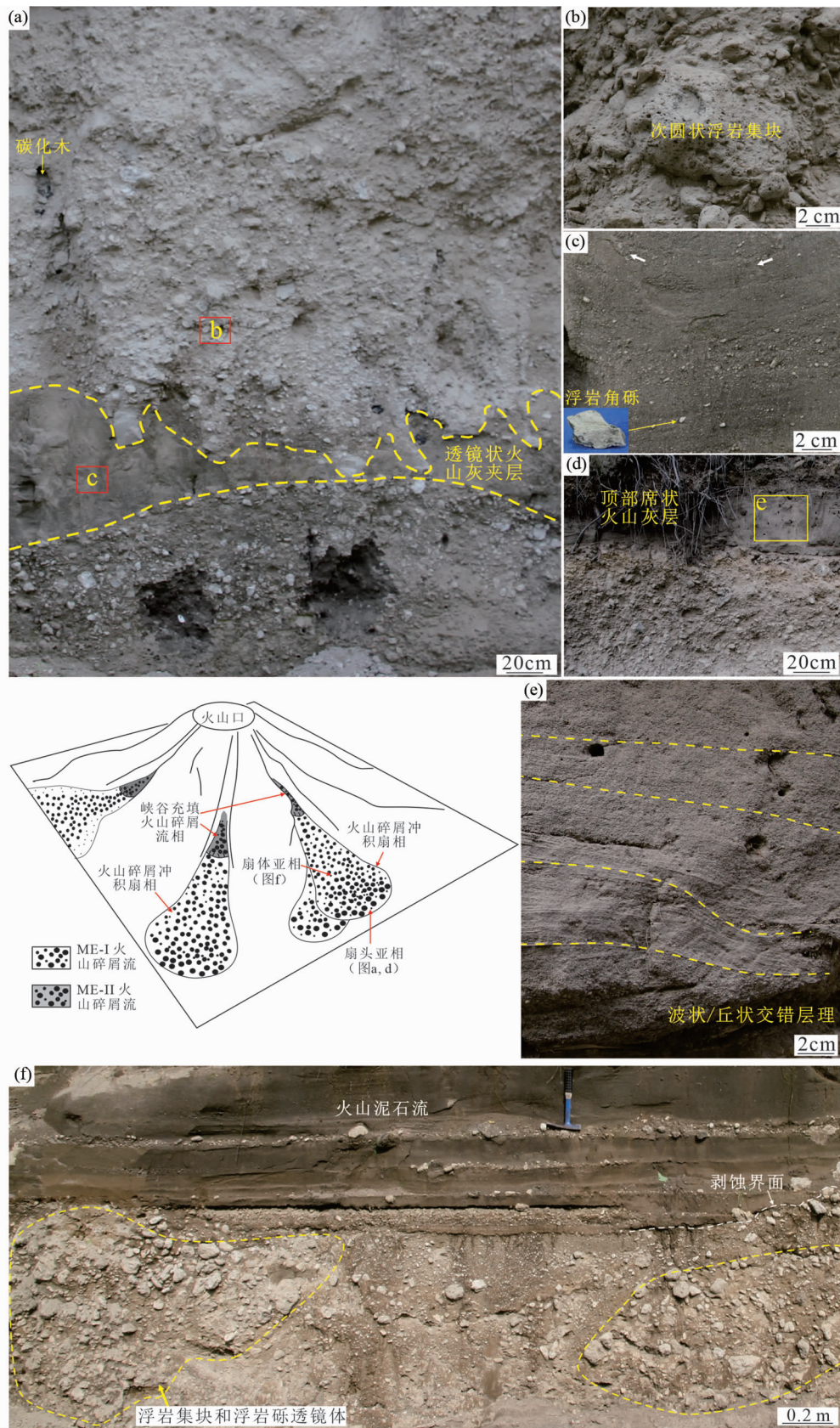
图8 长白山千年大喷发 ME- I 火山碎屑流冲击扇相典型堆积特征
