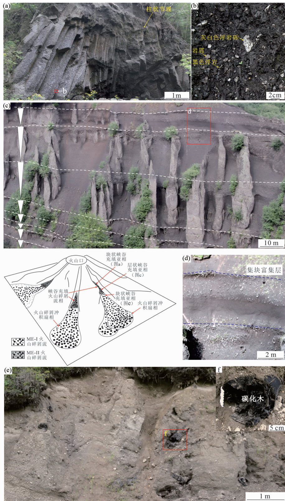
图6 长白山千年大喷发峡谷充填火山碎屑流相典型堆积特征
