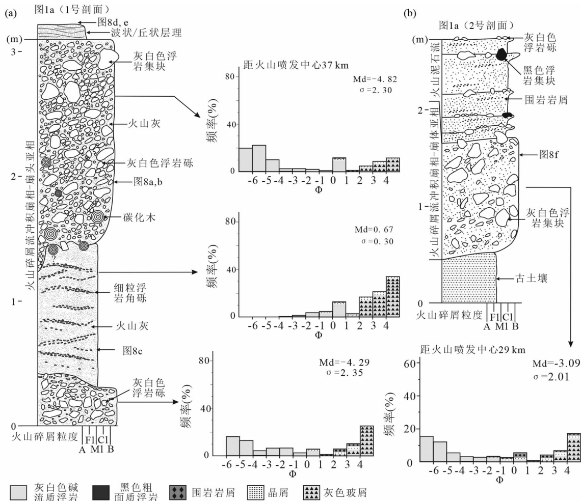
图9 长白山千年大喷发 ME- I 火山碎屑流冲击扇相典型垂向序列和粒度、成分特征
