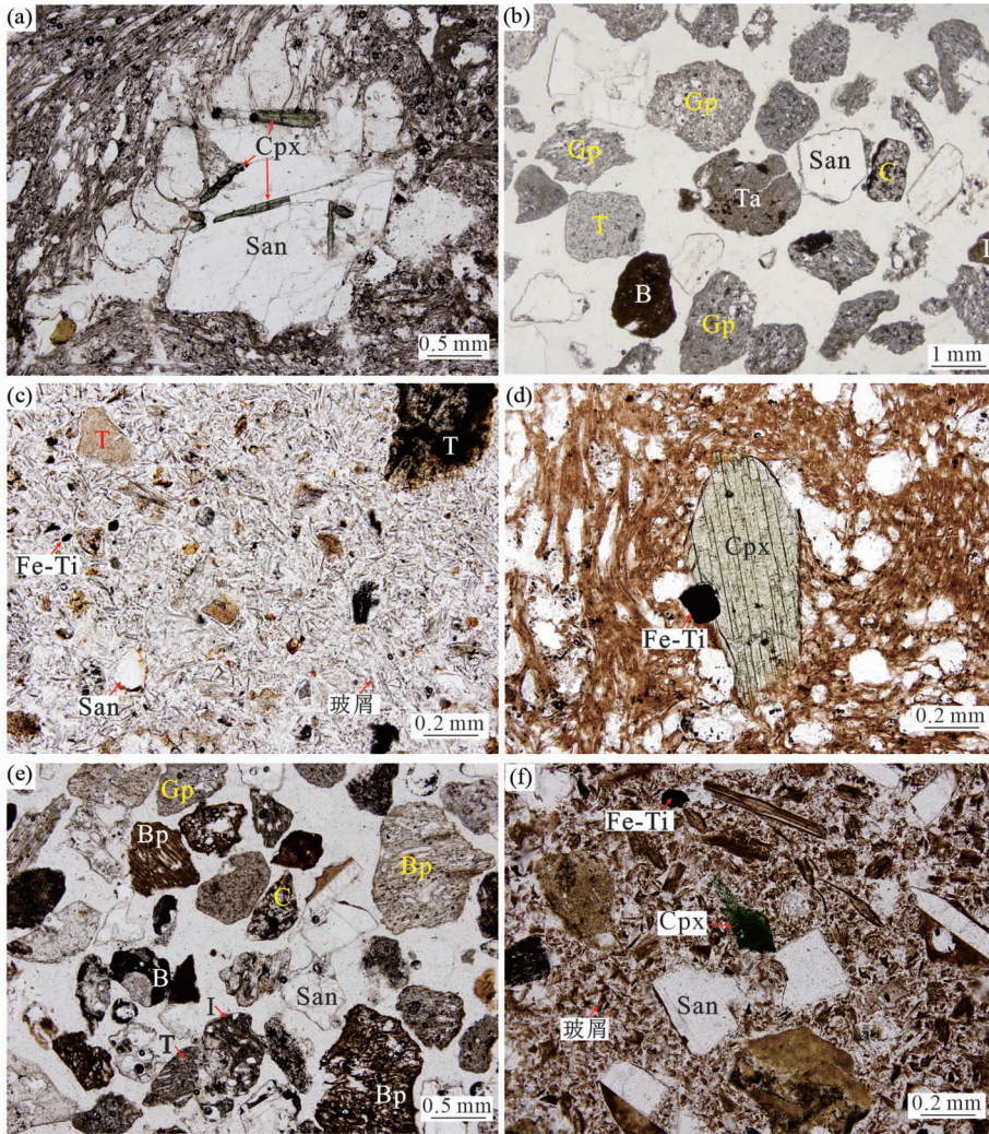
图3 长白山千年大喷发火山碎屑流堆积物典型显微照片
