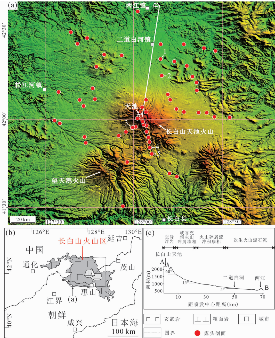
图1 长白山天池火山地理位置
