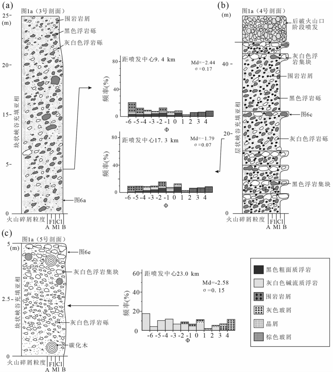
图7 长白山千年大喷发峡谷充填火山碎屑流相典型垂向序列和粒度成分特征
