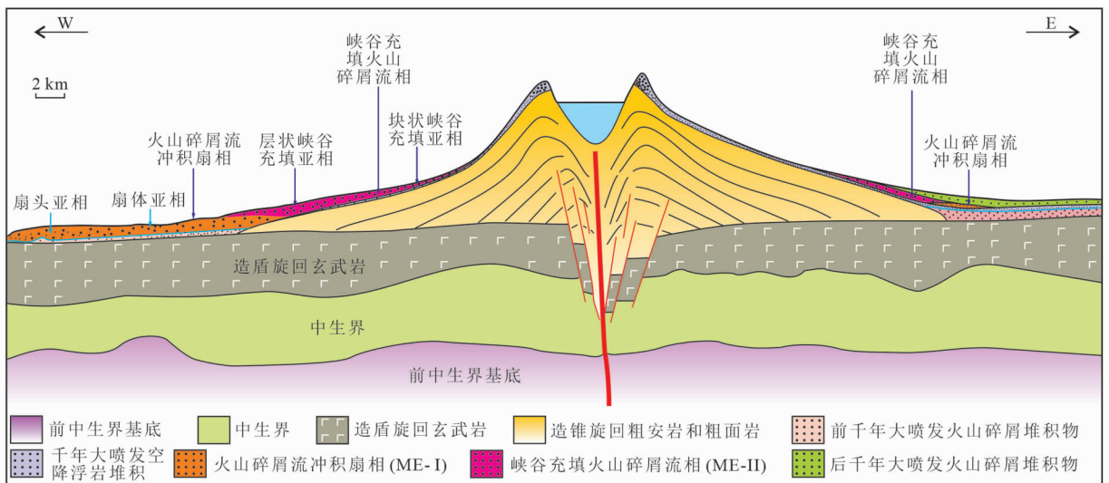
图5 长白山千年大喷发火山碎屑堆积物分布剖面图
