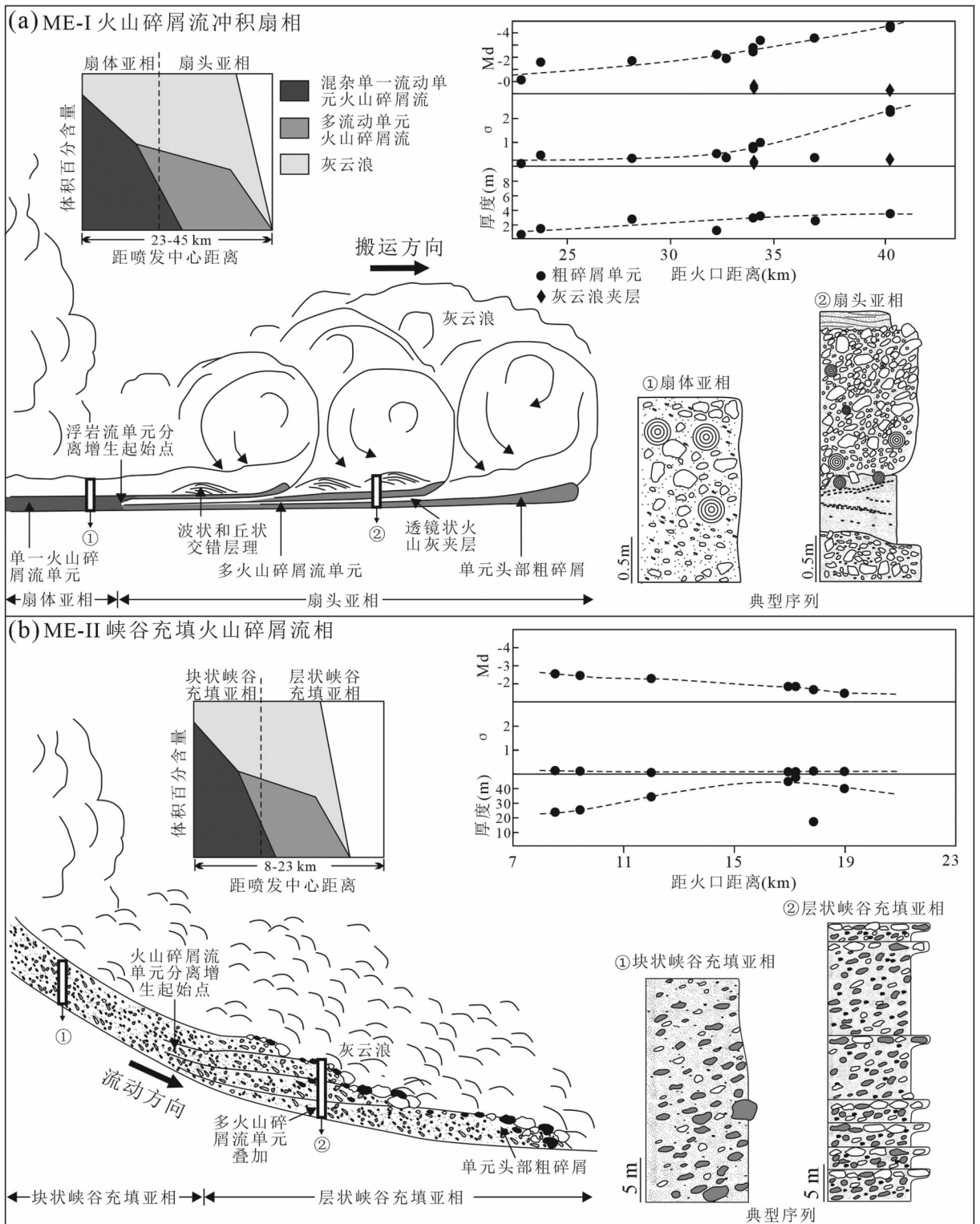
图 10 长白山千年大喷发火山碎屑流搬运和堆积过程及相模式
